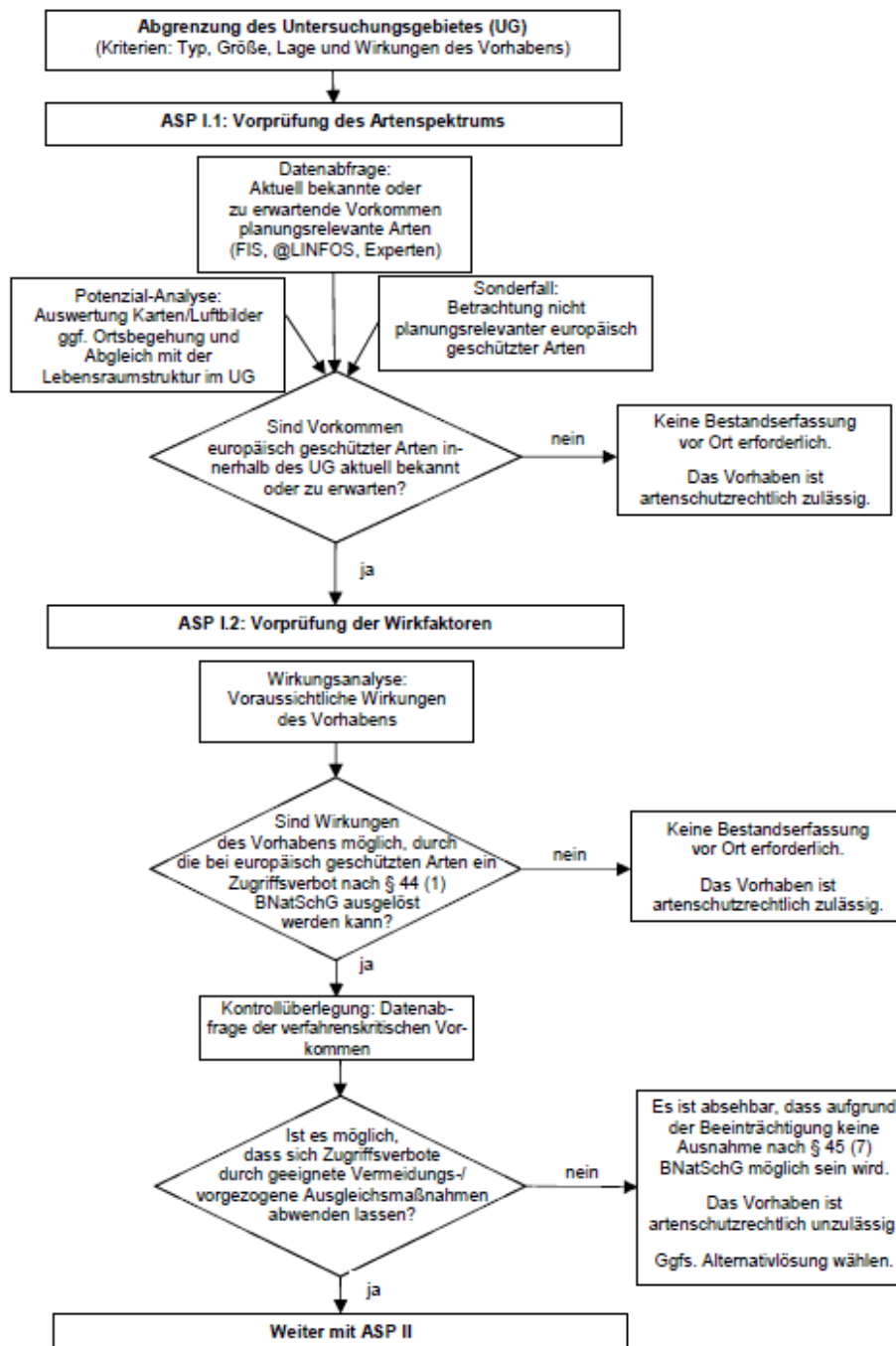
Abbildung 5: Ablaufschema der ASP Stufe I (aus: MKULNV 2010)
